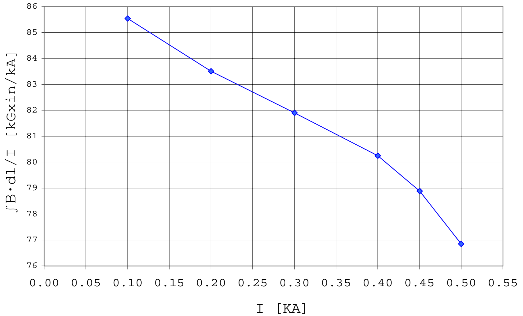
\int B \cdot dl / I vs I
