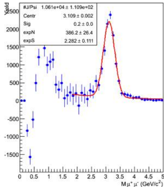
Dimuon Mass (GeV)
